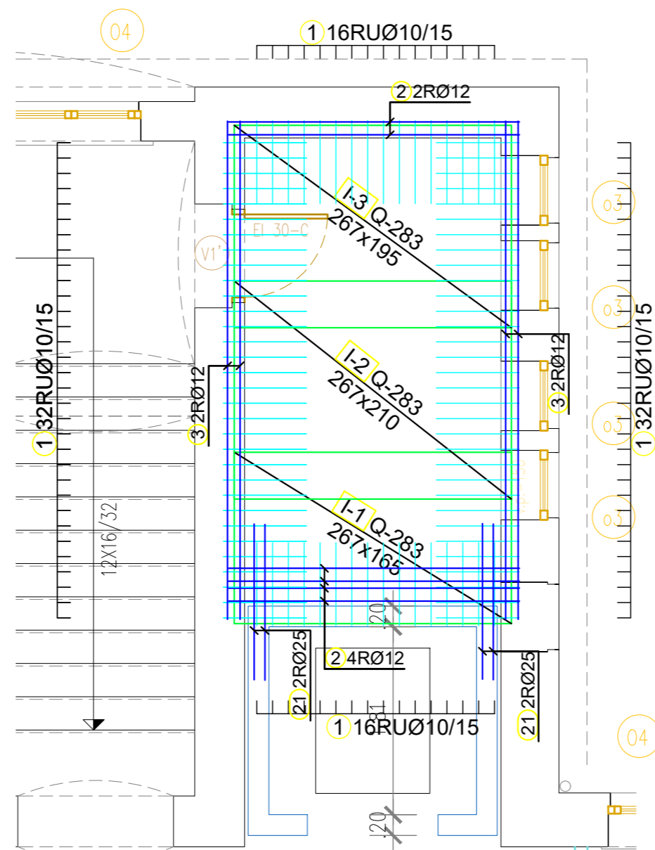
armatura SPODAJ
