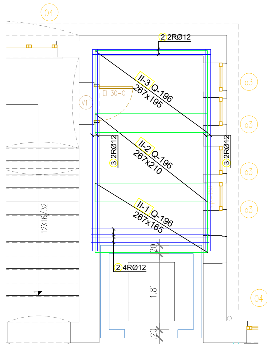
armatura ZGORAJ
